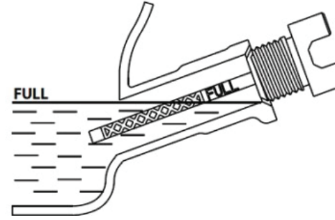
Resim-3 Yağ Seviyesi
